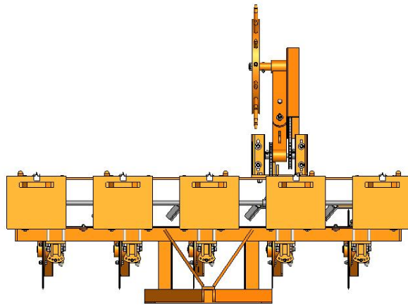
รูปที่ 17 ภาพด้านบนเครื่องหยอดเมล็ดพืชแบบ 5 แถว
