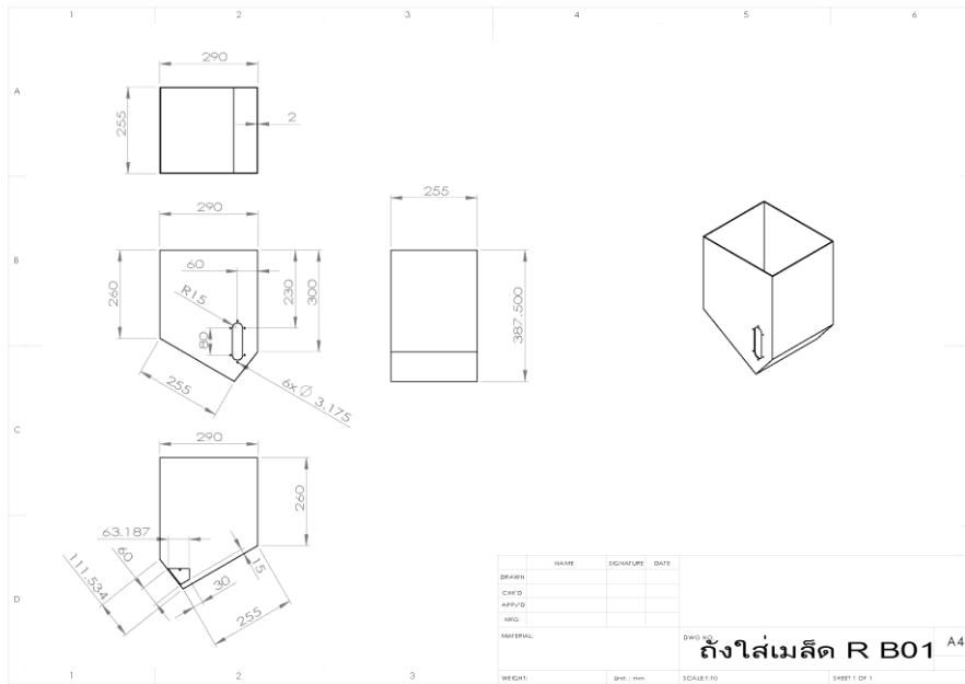
รูปที่ 5 ถังบรรจุเมลต์
