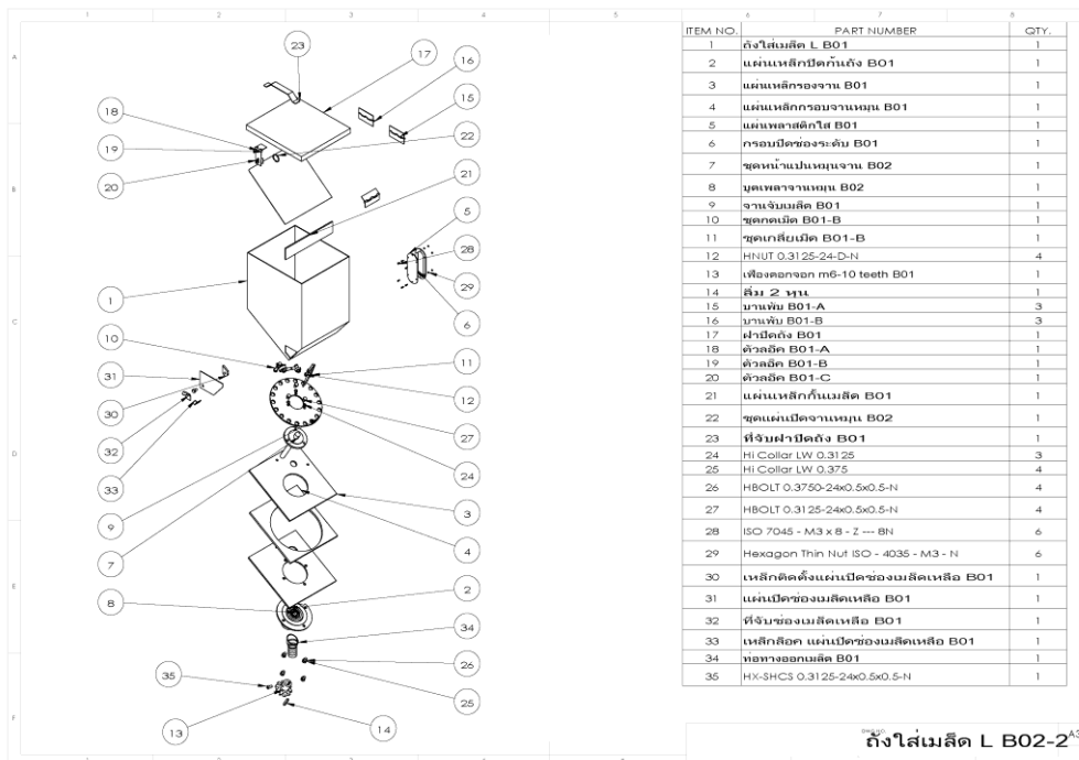
รูปที่ 6 องค์ประกอบของถังบรรจุเมลต์
