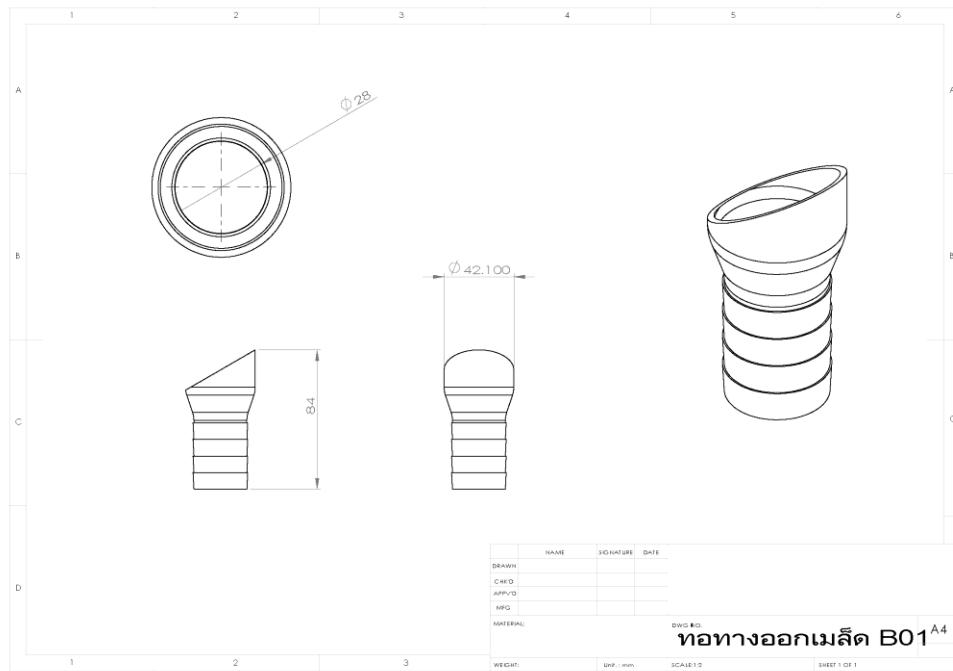
รูปที่ 8 ท่อส่งเมล็ด
