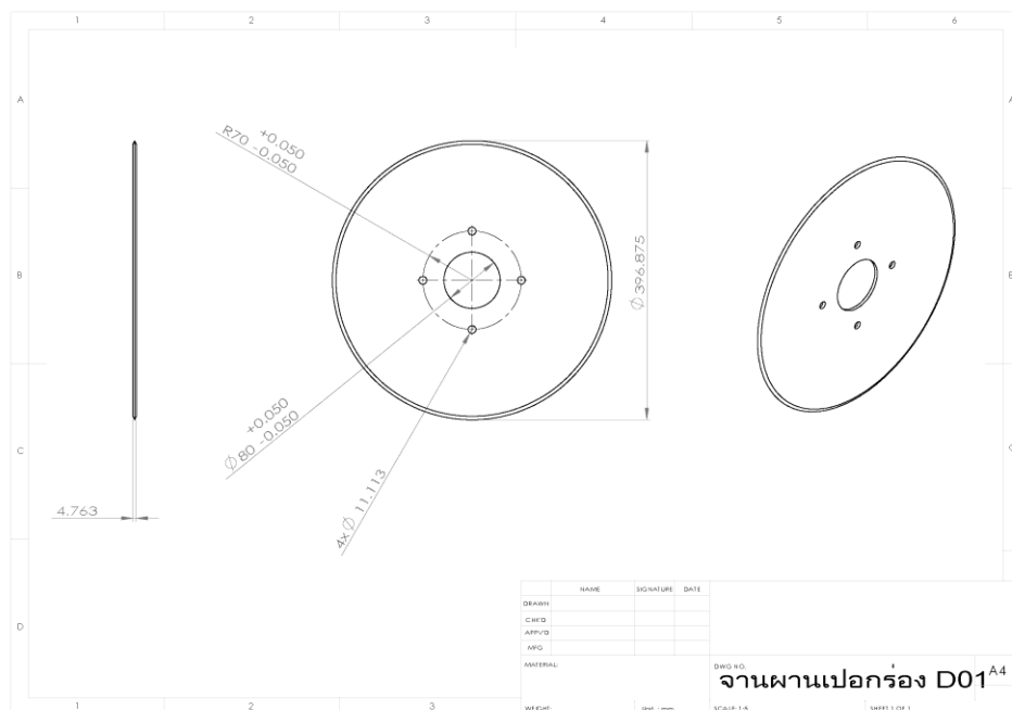
รูปที่ 9 ตัวเปิดร่อง
