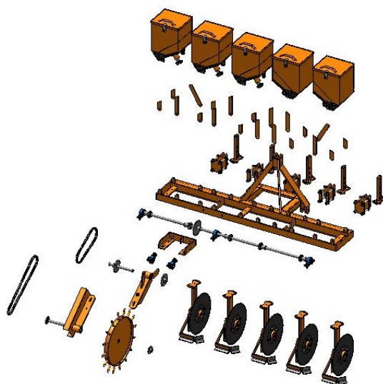
รูปที่ 19 ภาพส่วนประกอบของเครื่องหยอดเมล็ด
