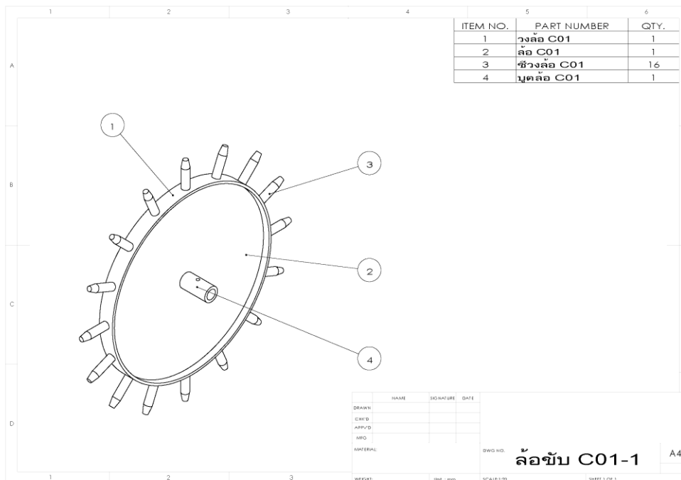
รูปที่ 13 ล้อขับ
