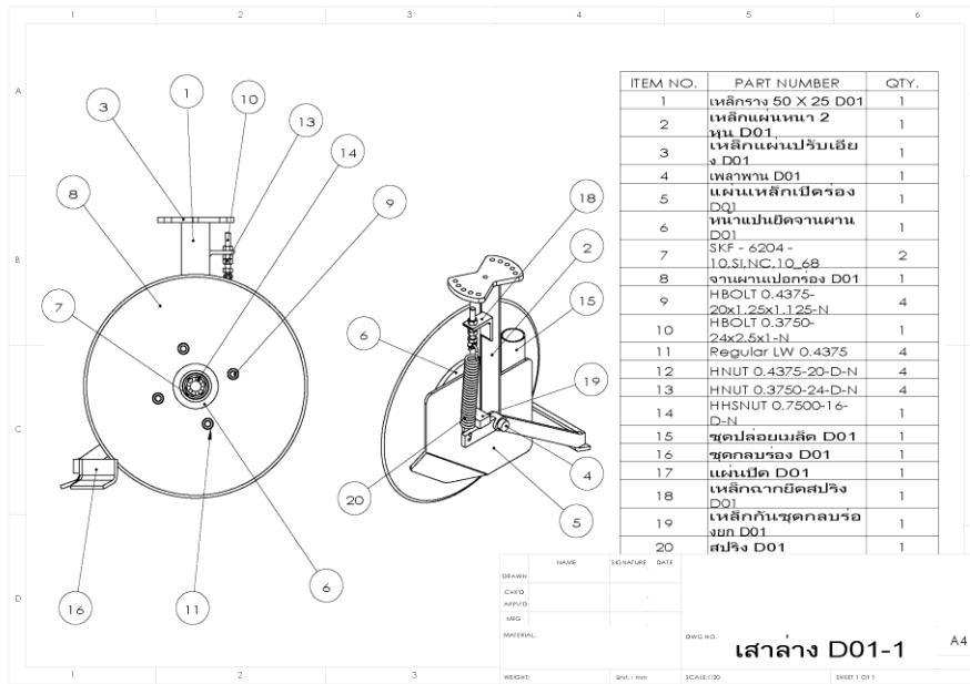
รูปที่ 10 องค์ประกอบของตัวเปิดร่อง
