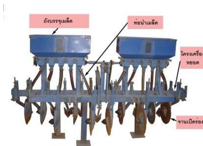
รูปที่ 4 เครื่องหยอดพวงดีตรถแทรกเตอร์ขนาดใหญ่
