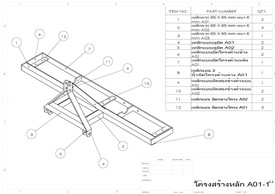
รูปที่ 14 ชุดโครงสร้างหลักของเครื่องหยอด
