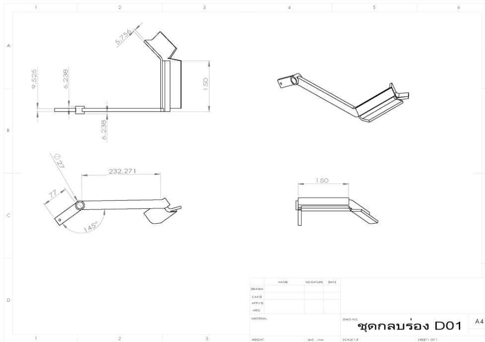
รูปที่ 11 อุปกรณ์กลบเมสิด
