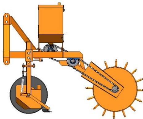
รูปที่ 18 ภาพด้านข้างเครื่องหยอดเมล็ดพืชแบบ 5 แถว
