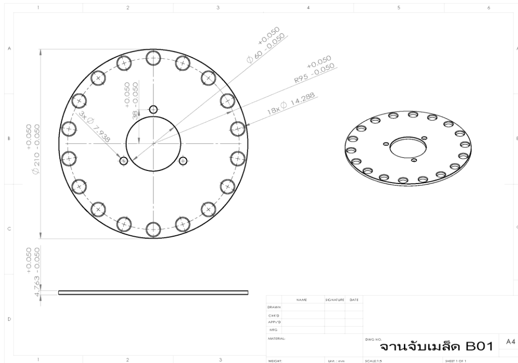
รูปที่ 7 ชุดแผ่นหยอดเมล็ด
