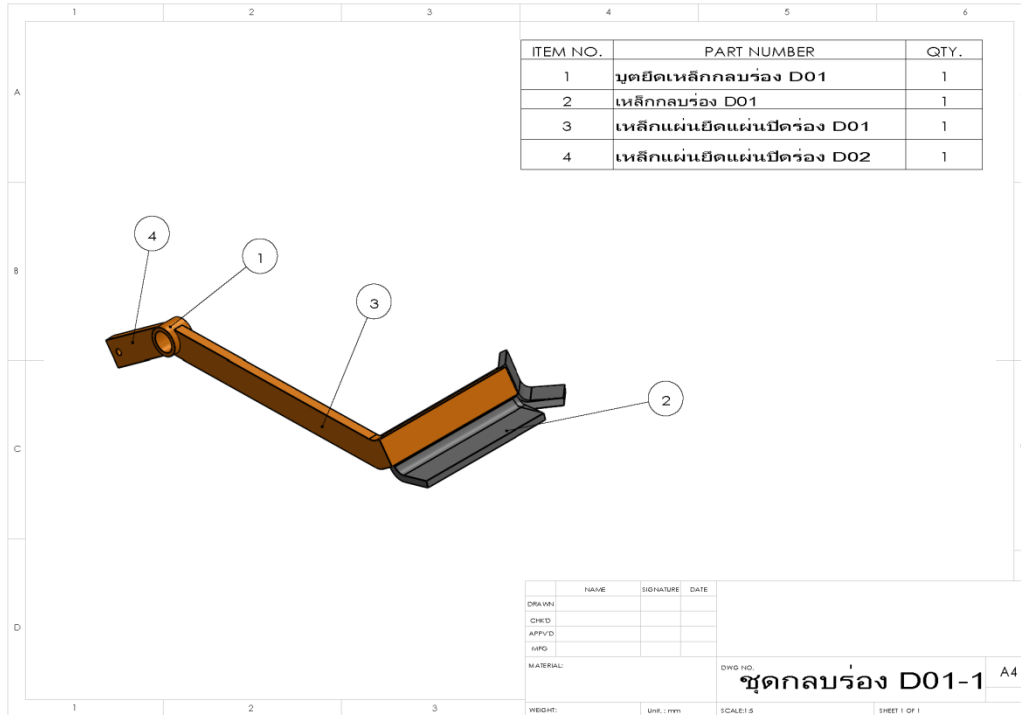
รูปที่ 12 องค์ประกอบของอุปกรณ์กลบเมล็ด
