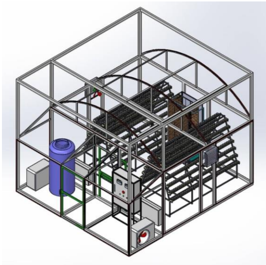
รูปที่ 8 โรงเรือนกระตุ้นตาดอกดำเนินการก่อสร้างที่ ศวศ.เชียงใหม่
