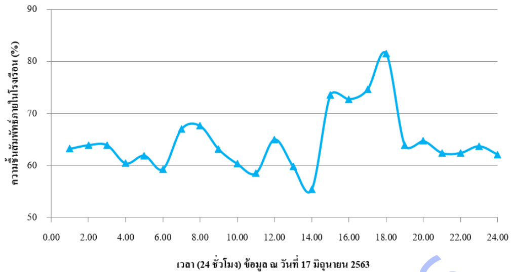
รูปที่ 6 ตัวอย่างข้อมูลความชื้นสัมพัทธ์ภายในโรงเรือน
