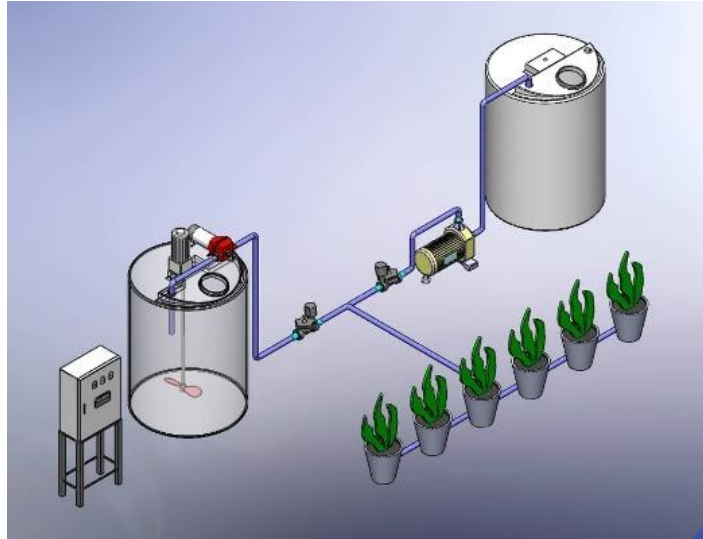
รูปที่ 18 ระบบการให้น้ำละอูย
