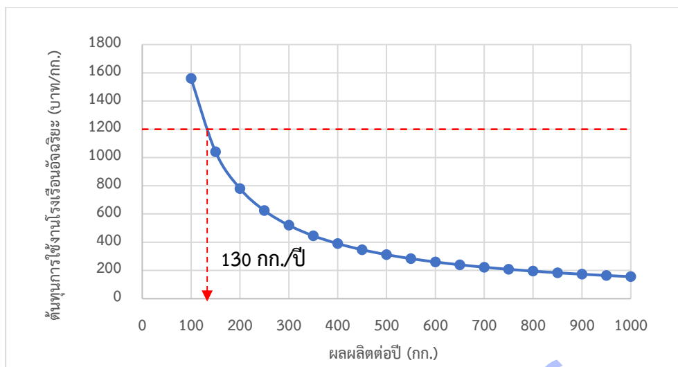
รูปที่ 29 ความความสัมพันธ์ระหว่างต้นทุนการใช้งานโรงเรือนอัจฉริยะต่อปริมาณผลผลิตต่อปี
