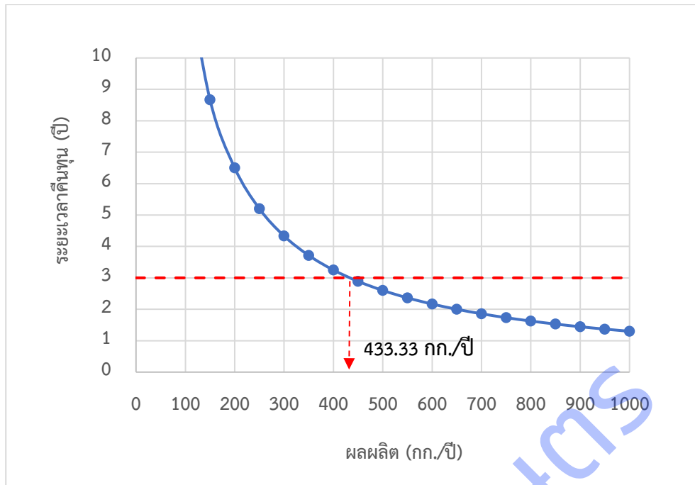
รูปที่ 30 ความความสัมพันธ์ระหว่างระยะเวลาการลงทุนของโรงเรือนอัจฉริยะกับผลผลิตต่อปี
