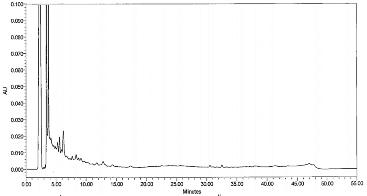
รูปที่ 30 HPLC chromatogram ของสารสกัดจากเอื้องแปรงสีฟัน ( D. secundum )
