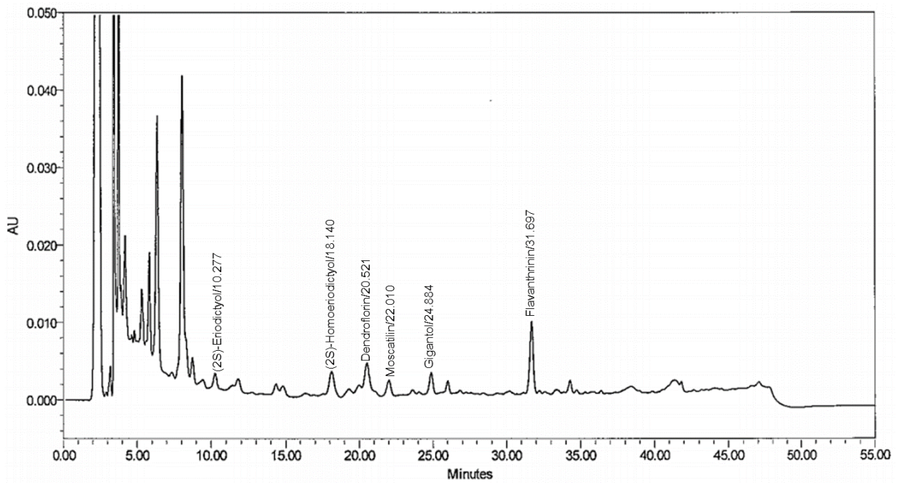
รูปที่ 35 HPLC chromatogram ของสารสกัดจากเองสายน้ำเขียว ( D. crepidatum )
