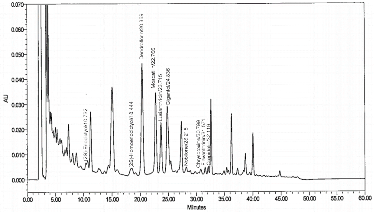
รูปที่ 12 HPLC chromatogram ของสารสกัดจากหวายตะมอย ( D. crumenatum )
