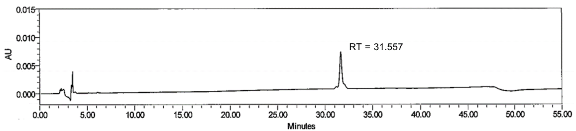
รูปที่ 10 HPLC chromatogram ของ Crepidatin Reference Standard (20 \mu\text{g/mL} )
