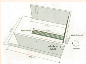
ภาพที่ 2 โรงเรือนผลิตปุ๋ยหมักแบบเติมอากาศ ขนาด 3x3x1.5 เมตร
