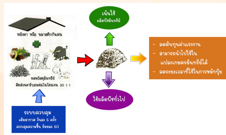
ภาพที่ 3 แนวผังกระบวนการผลิตปุ๋ยหมักแบบเติมอากาศ
