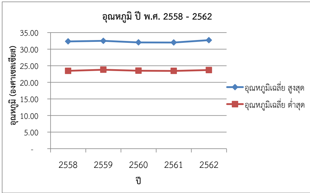
ภาพผนวกที่ 2 อุณหภูมิเฉลี่ยสูงสุด - ต่ำสุด ภายในศูนย์วิจัยพืชสวนชุมพร ปี พ.ศ. 2558 - 2562
